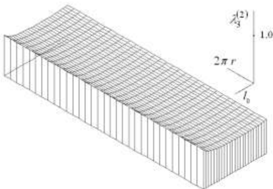
Рис. 3. Утонение во внутренней оболочке \Omega_2
