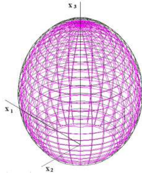
Рис. 5. Объем оболочки V = 56.85 \text{ м}^3 при давлении p^{(2)} = p_{кр}^{(2)} = 0.5015625
