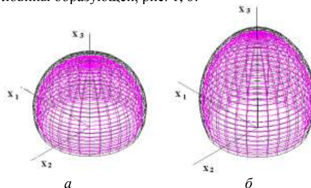
Рис. 1. Форма оболочек при времени \tau = 0 (а) и \tau = 1.61 (б)
