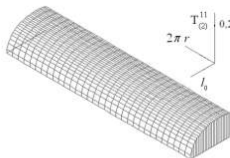
Рис. 2. Осевые поверхностные натяжения на оболочке \Omega_2
